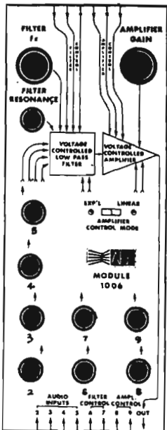
ARP FiltAmp Module 1006
