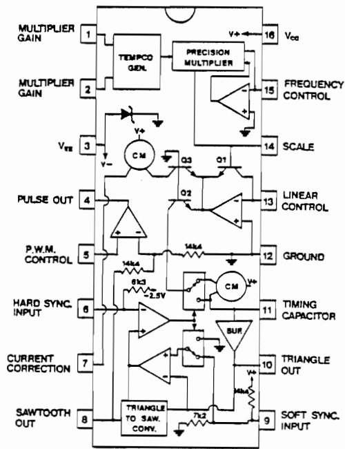
FIGURE 3. CEM 3340 IC
